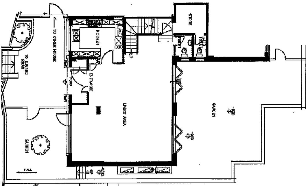
G/F Layout
